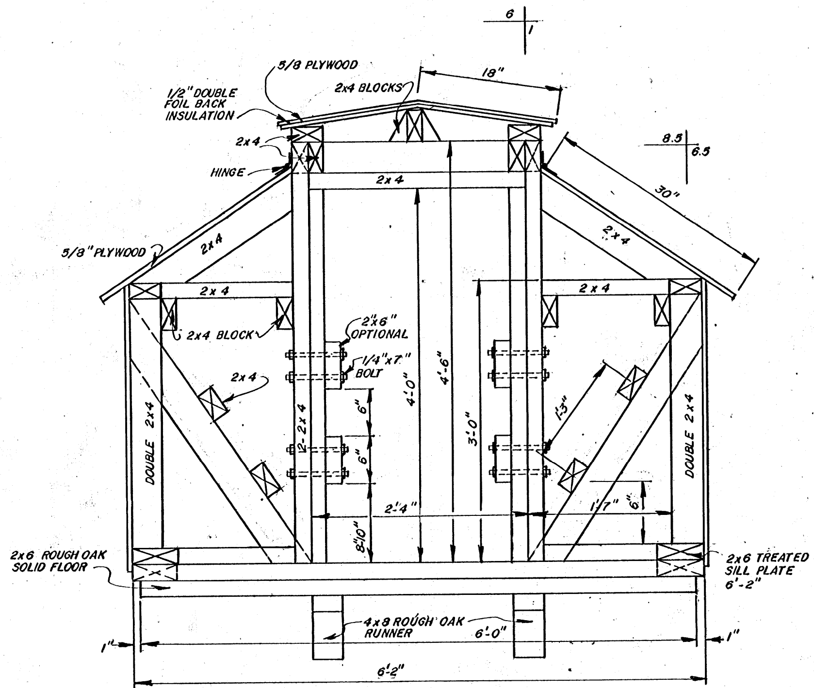
END VIEW Scale: 1" = 1'-0"
